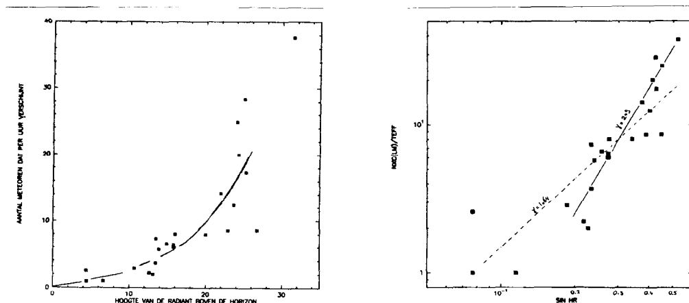
Figuur 3-8: Uit de figuur volgt: \gamma = 2.2 \pm 0.7 .
